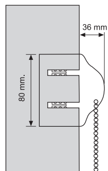
INSTALACIÓN A PARED FACE FIX
